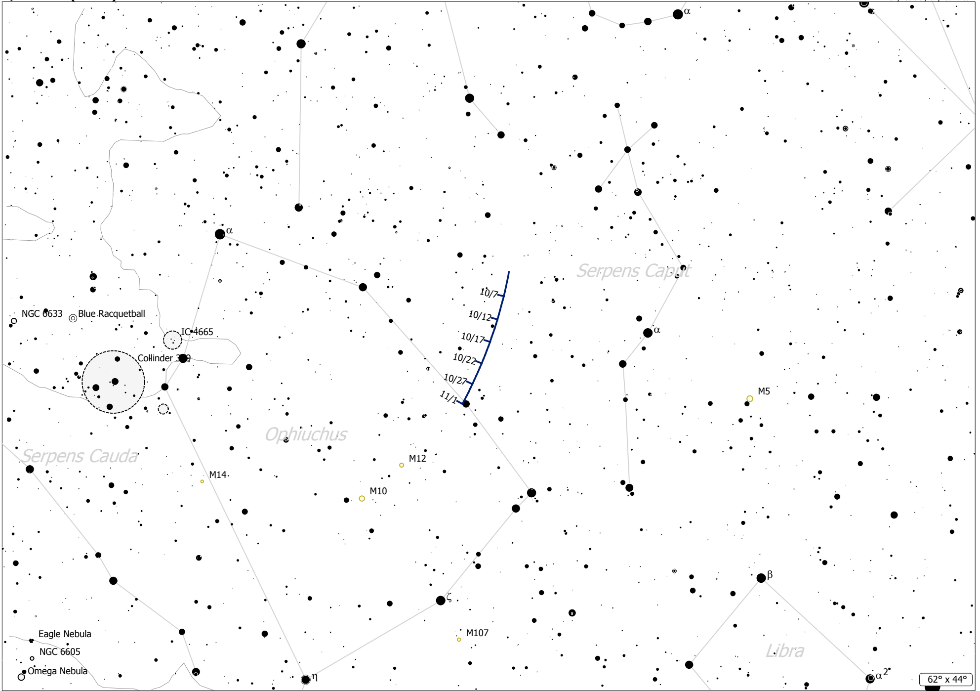
C/2017 M4 (ATLAS) (Comet) Magnitude: 14.14 Coma Diameter: 48" SBr: 22.3 Mag/arcsec 2 Earth
