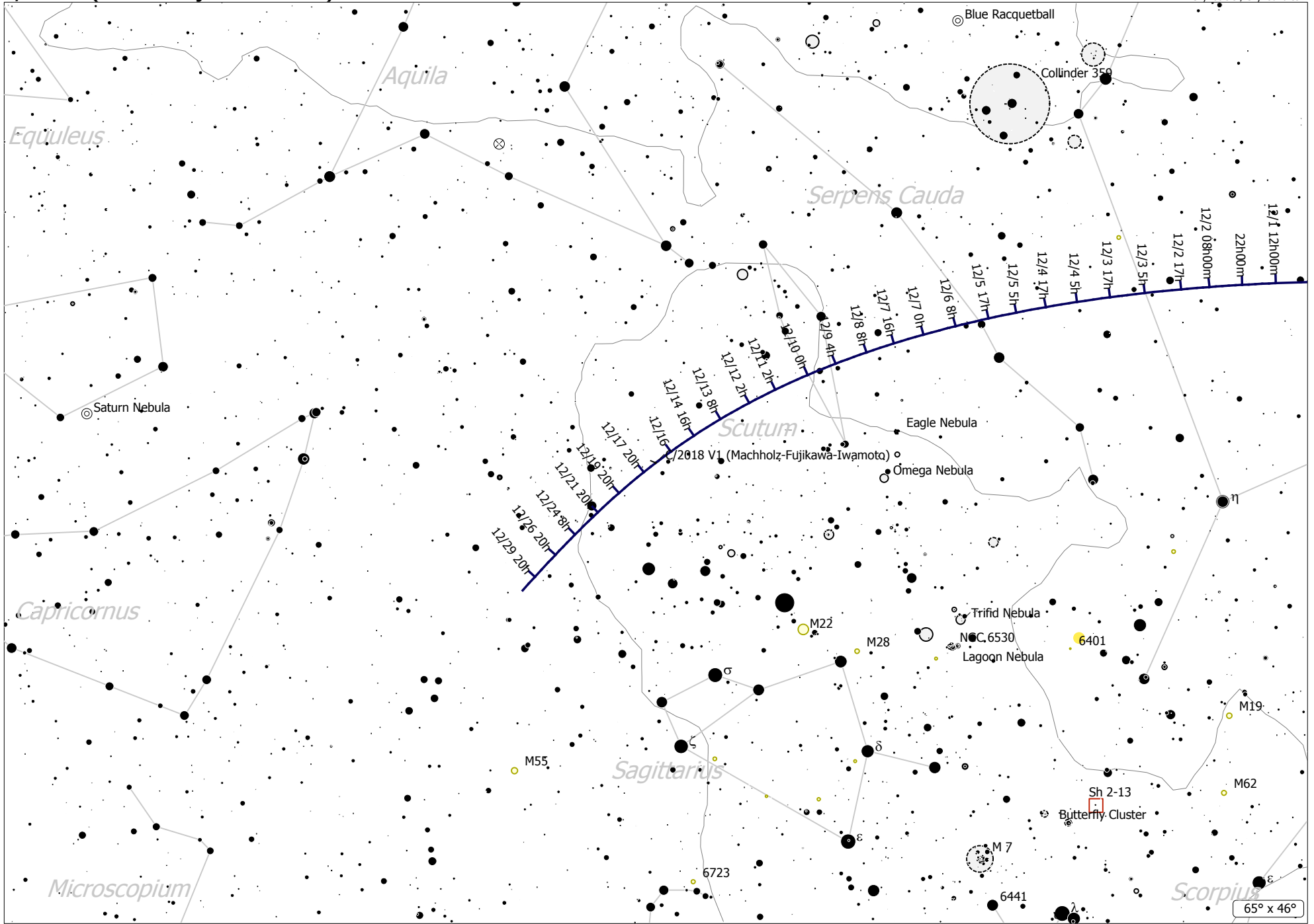
C/2018 V1 (Machholz-Fujikawa-Iwamoto) (Comet) Magnitude: 7.90 Coma Diameter: 4.3' SBr: 19.7
