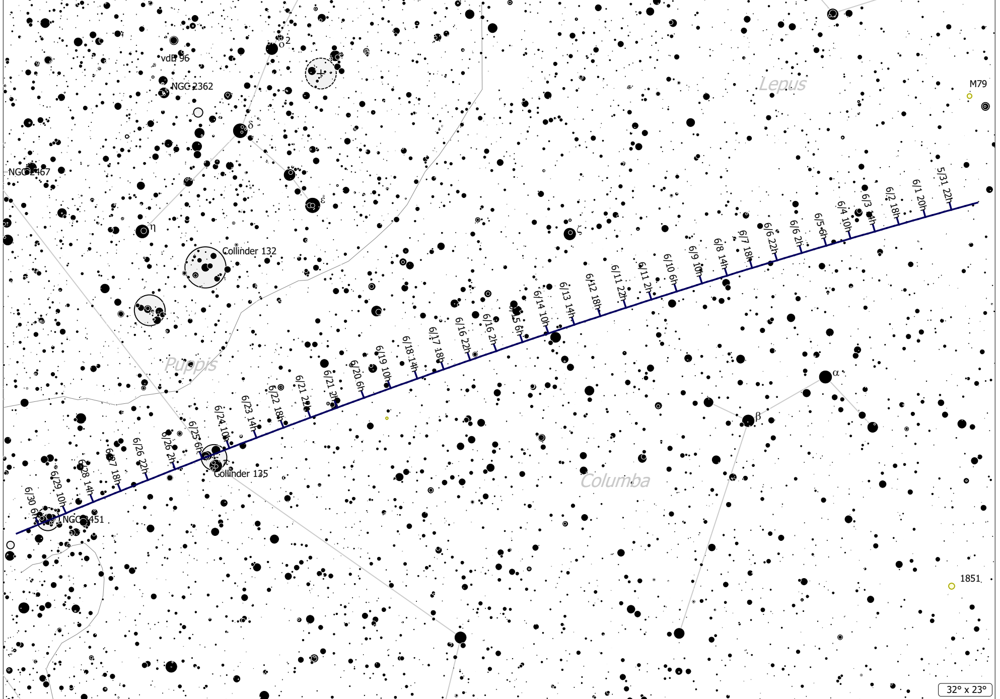
C/2018 W1 (Catalina) (Comet) Magnitude: 11.19 Coma Diameter: 4.7' SBR: 23.2
