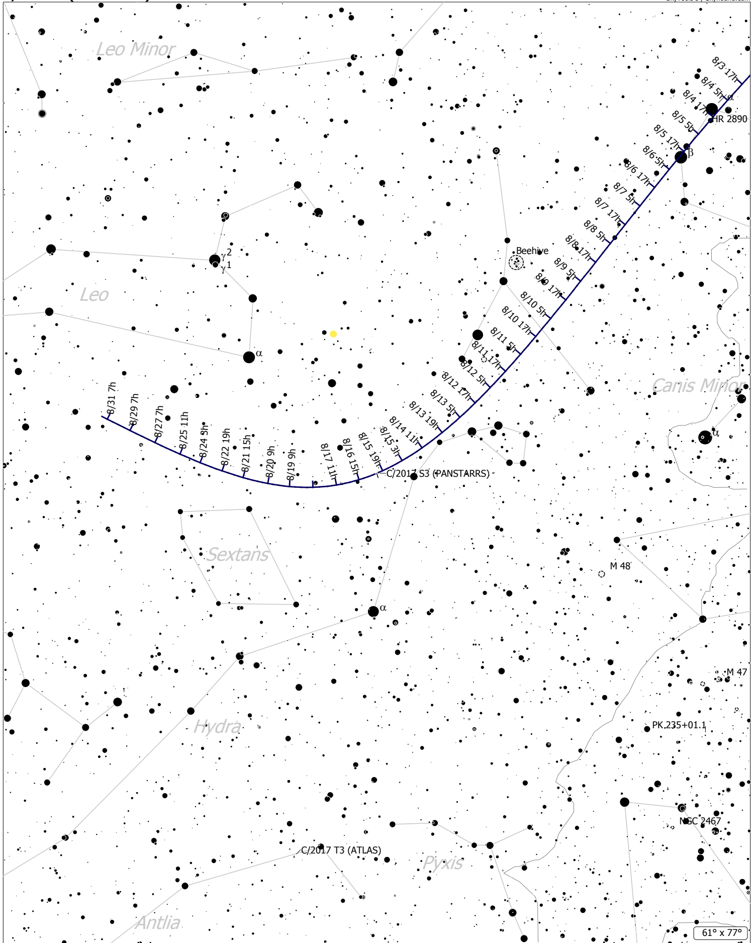
C/2017 S3 (PANSTARRS) (Comet) Magnitude: 3.52 Coma Diameter: 4.5' SBr: 15.4 Mag/arcsec 2 Earth
