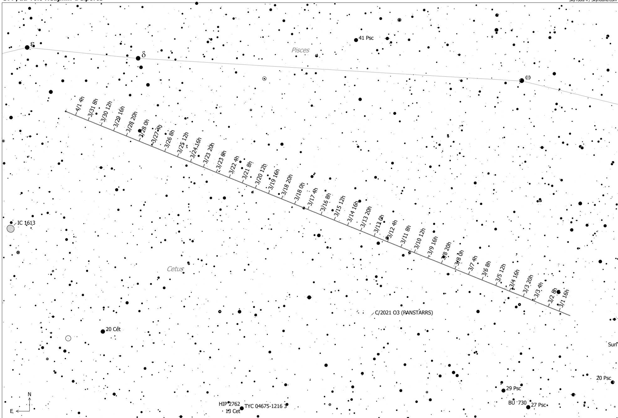
57P/du Toit-Neujmin-Delporte (Comet)
